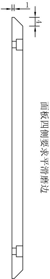
2-2剖视图
